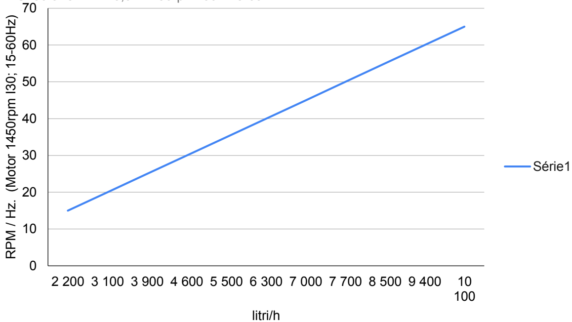
AS100 3Bar - kW 3,0 - 1450rpm I30 - 15-65Hz
